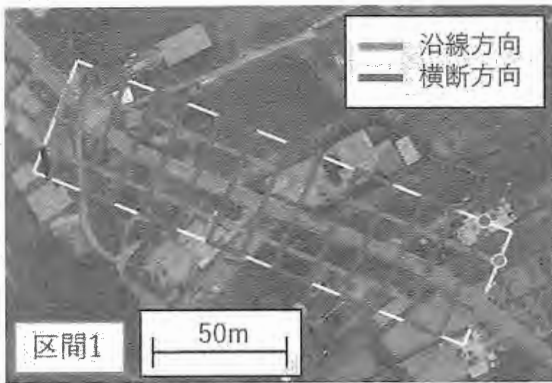
図-2 飛行経路の例 (区間1; 撮影高度 50m; 天底角 0^\circ )。以下, ⑤は撮影開始地点, ⑥は撮影終了地点を示す。
