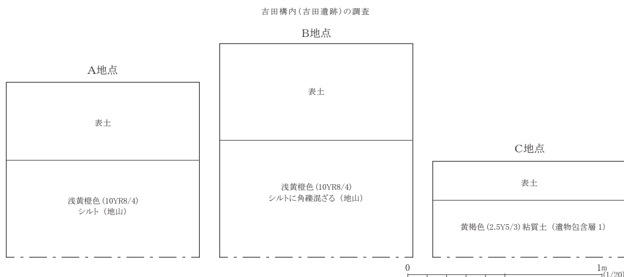
図 37 A～C地点土層断面柱状図
