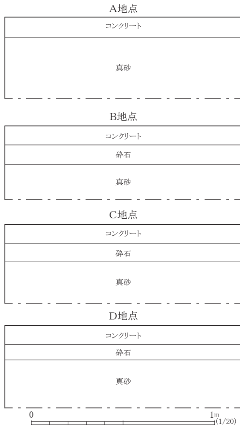
図 51 A～D地点土層断面柱状図
