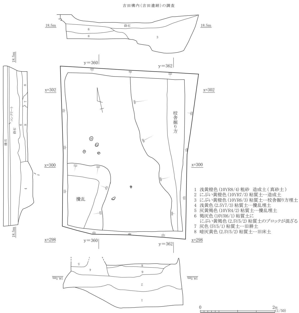
図7 第2調査区平面図・断面図
