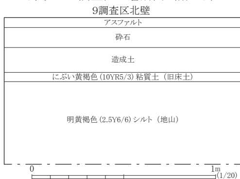
図45 9調査区土層断面柱状図
