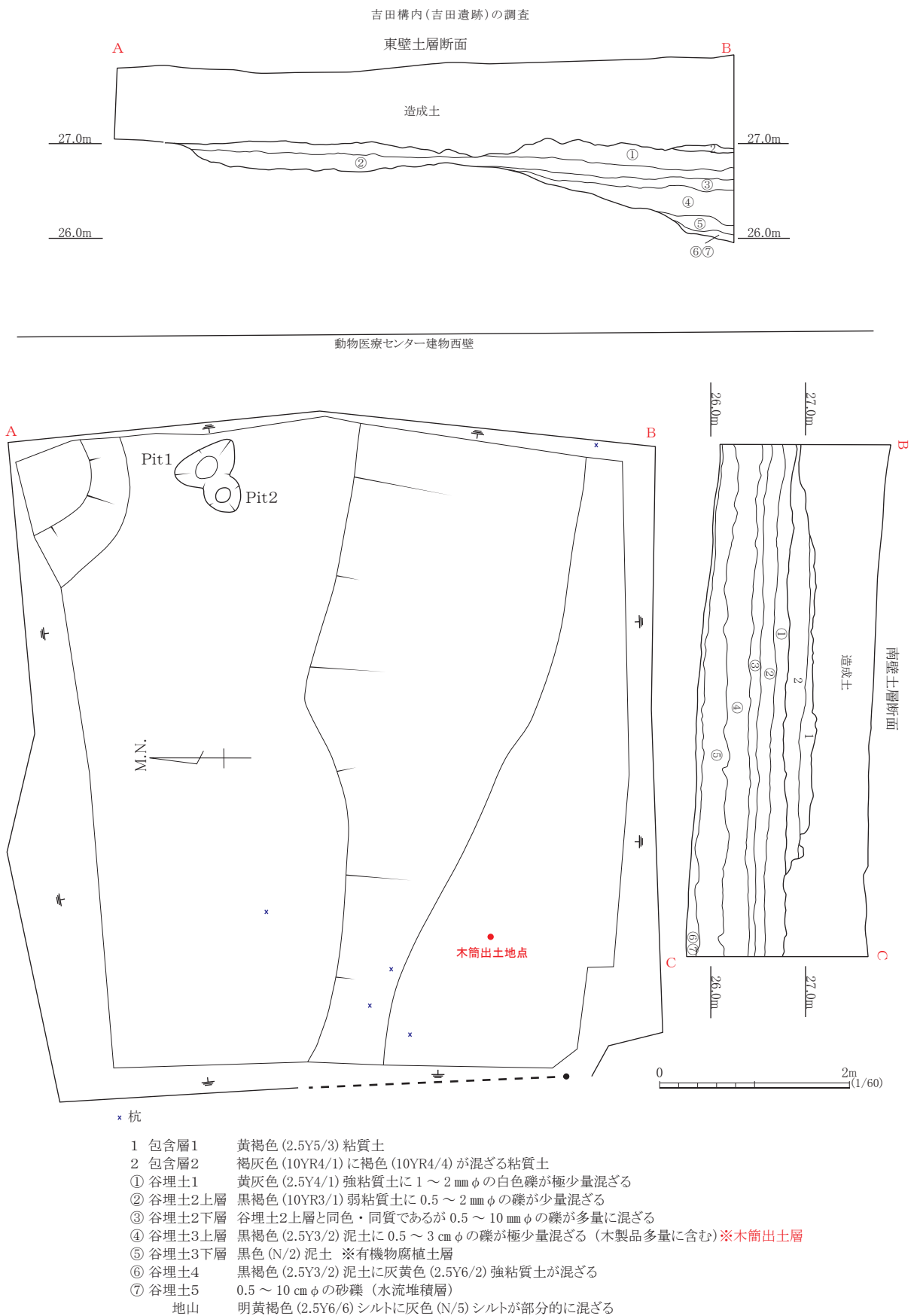
図 17 調査区平面図・断面図
