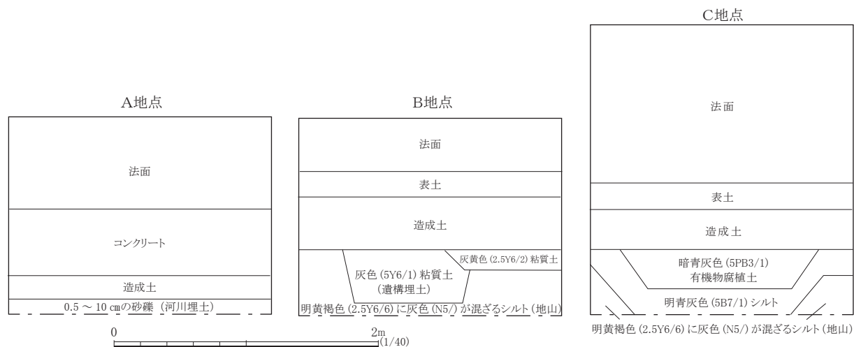
図 43 A～C地点土層断面柱状図
