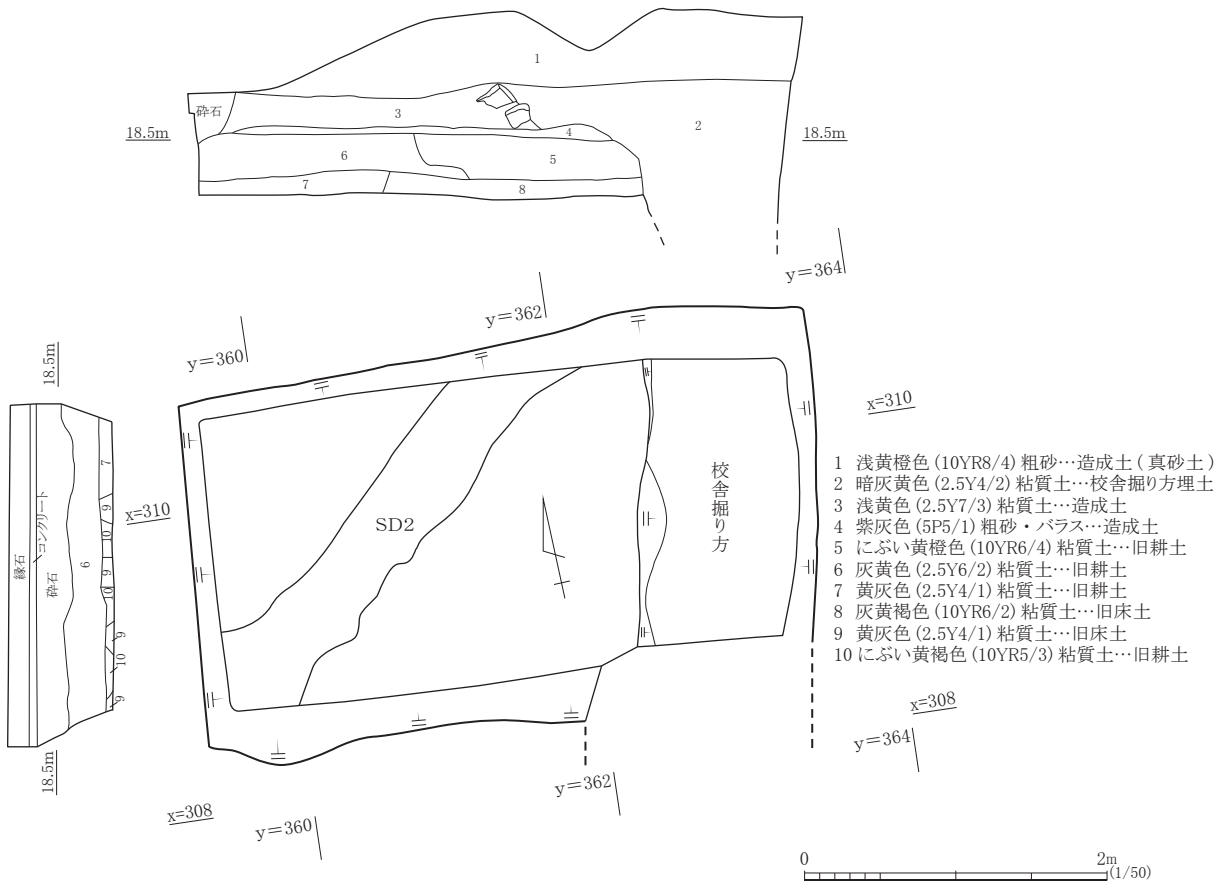
図9 第4調査区平面図・断面図
