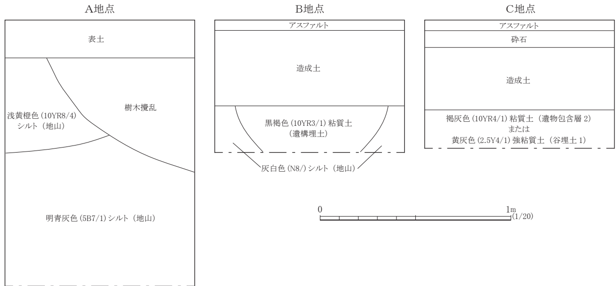
図 34 A～C地点土層断面柱状図
