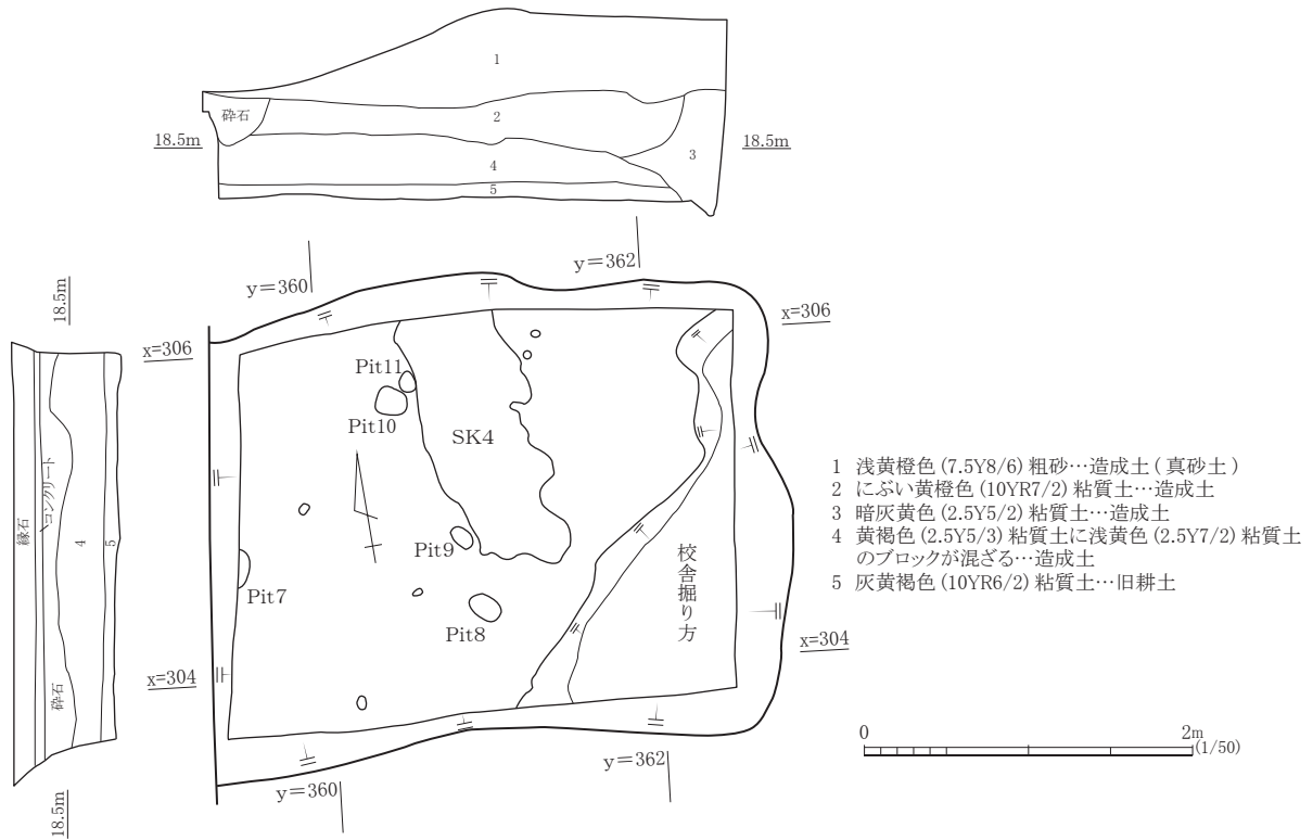
図8 第3調査区平面図・断面図
