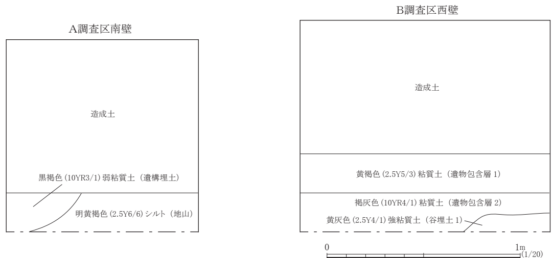
図 31 A・B調査区土層断面柱状図
