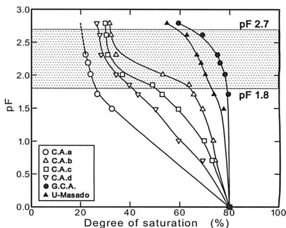
図-2 各試料の水分特性曲線
