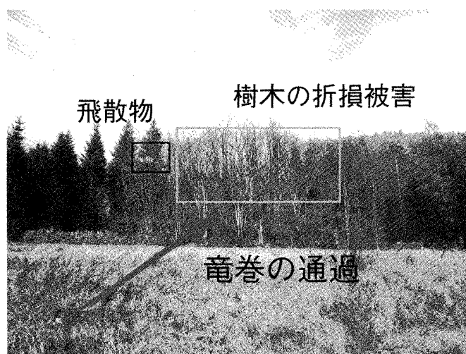
写真8 竜巻の通過地点 (2006年11月9日撮影)
