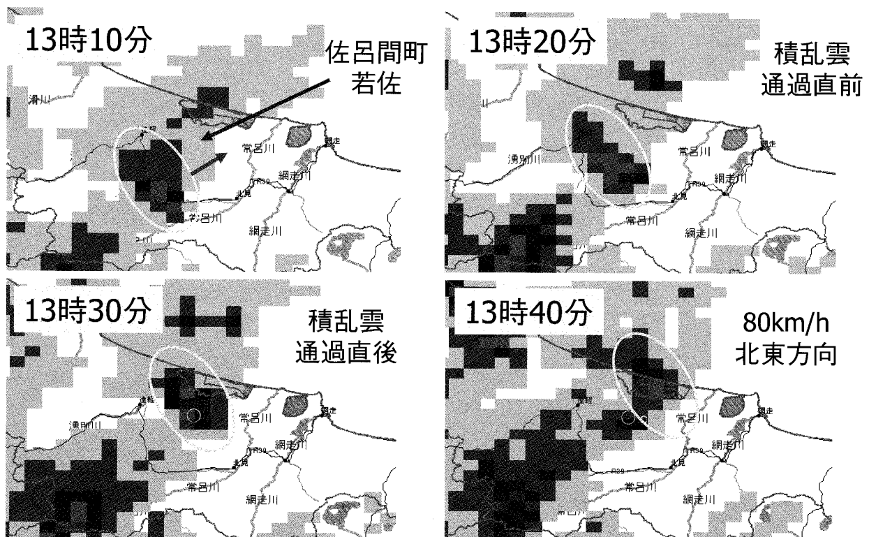
図5 レーダ雨量図 (2006年11月7日)
