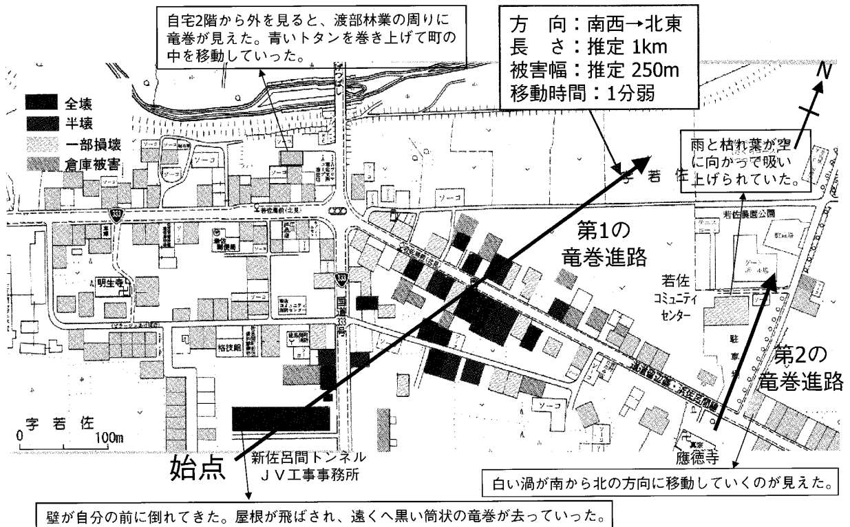
図8 佐呂間町若佐地区における建物被害の状況 (佐呂間町提供, 2006年11月10日, ほぼ確定値)
