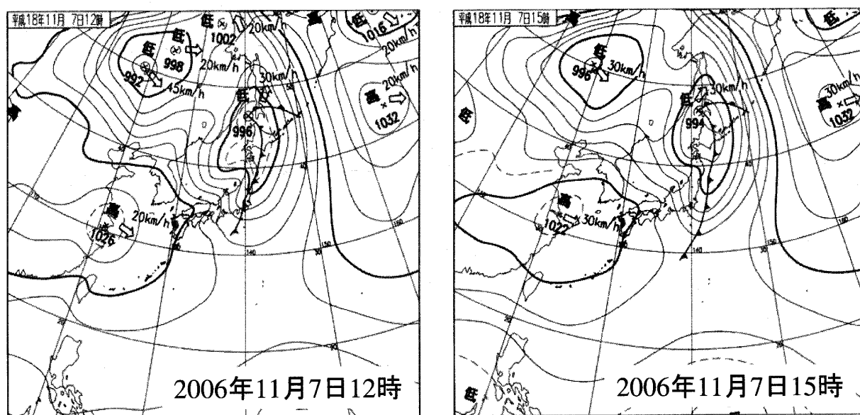
図3 竜巻発生前後の地上天気図
