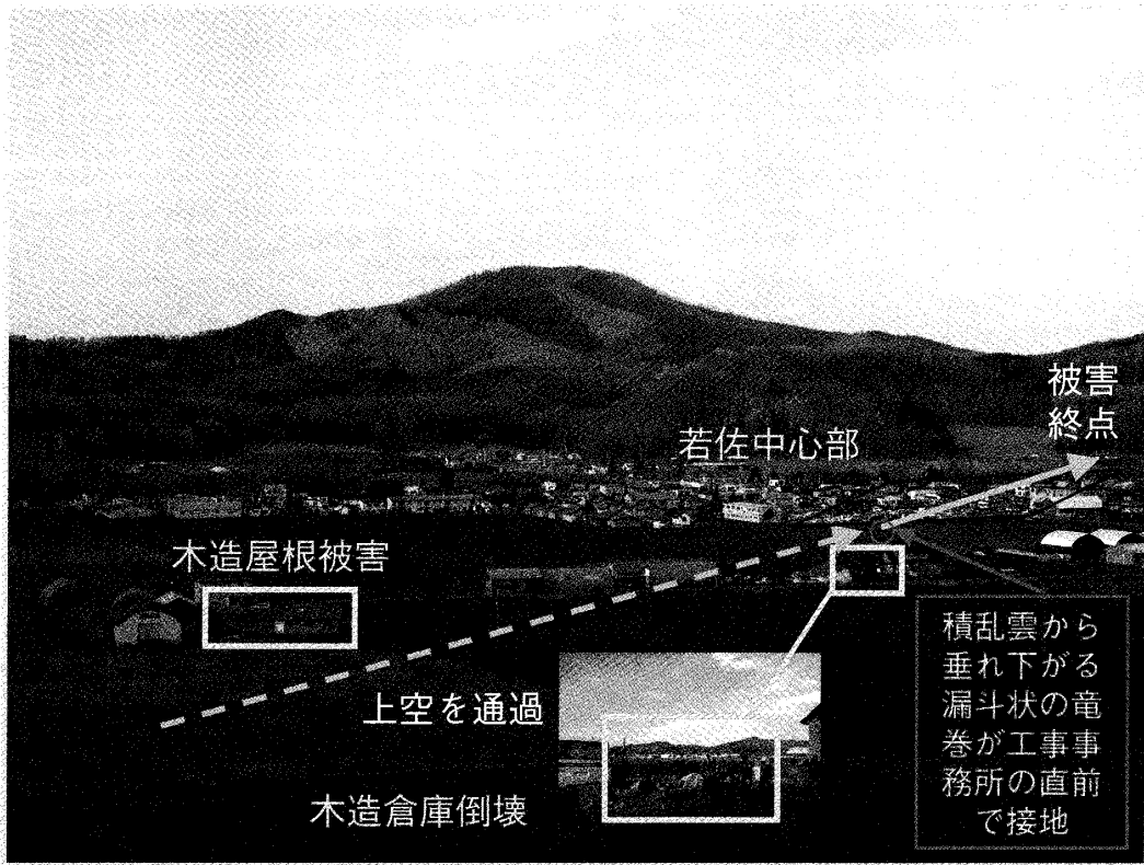
写真2 若佐地区中心部までの竜巻の経路 (2006年11月9日撮影)
