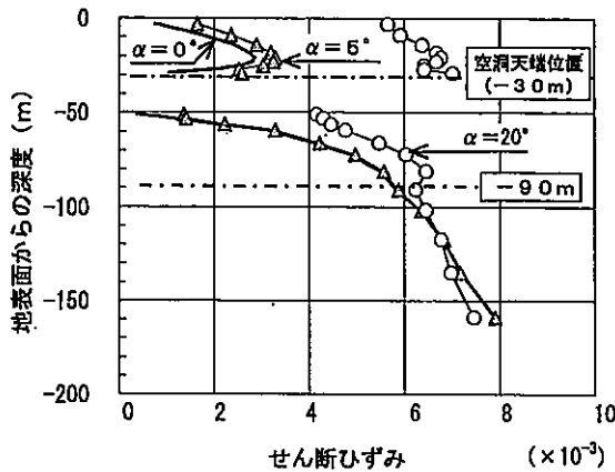
図-11 空洞中心軸上のせん断ひずみの分布
