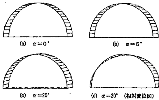
図-10 空洞の上下最大相対変位発生時の変位図
