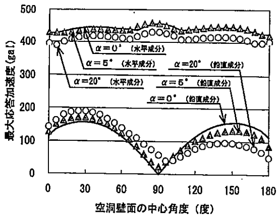
図-7 空洞周辺岩盤の最大応答加速度の分布
