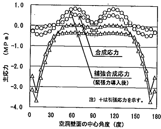
図-17 ロックアンカーにより緊張力を導入する前後の合成応力の比較
