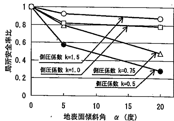
図-16 各側圧係数の \alpha = 0^\circ における地震時最小局所安全率を基準にした局所安全率比
