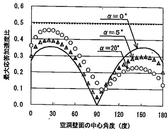
図-9 水平成分に対する鉛直成分の最大応答加速度比
