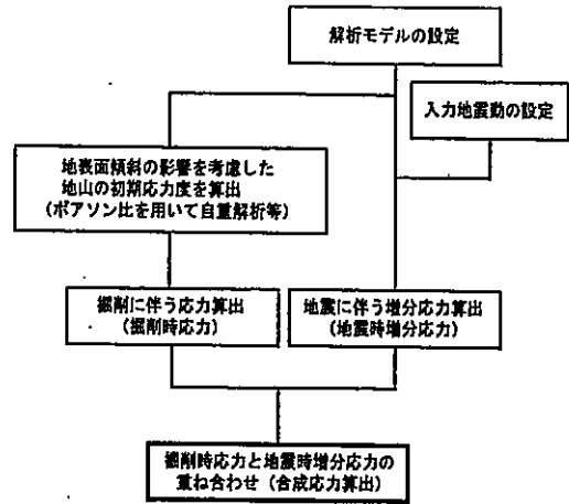
図-5 合成応力の算出手順
