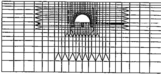
図-4 解析モデル (モデル I)
