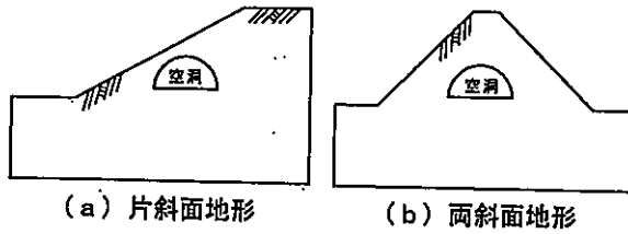
図-1 地表面地形の不整形
