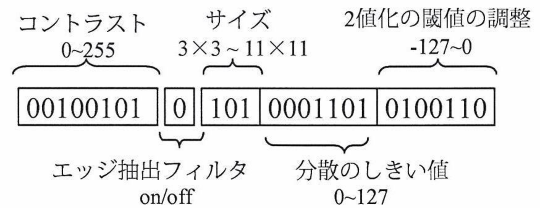
図-3 遺伝子のコーディング
