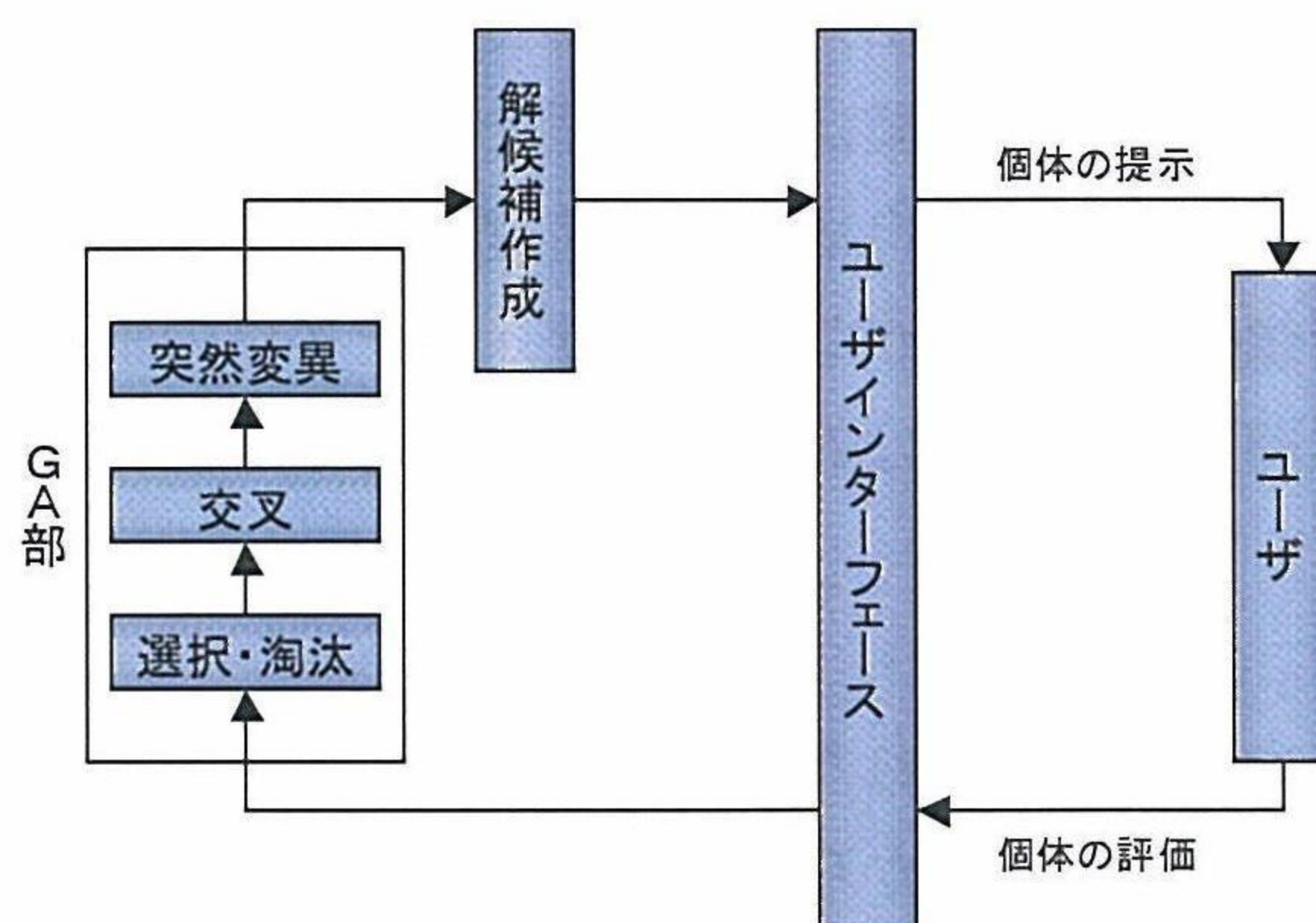
図-1 対話型 GA の基本フロー
