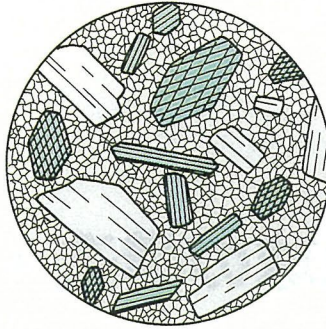
完晶質斑状組織 (半深成岩)
