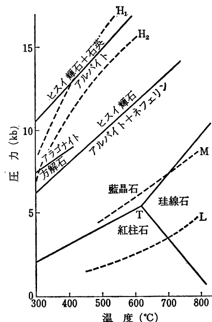
図5 紅柱石－珪線石－藍晶石の安定領域と変成相系列。L:低圧型，M:中圧型，H:高圧型。(都城秋穂・久城育夫，1977，岩石学 III，共立全書による)
