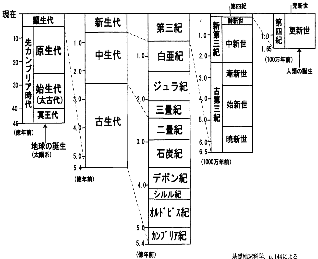
図2 地質年代区分
