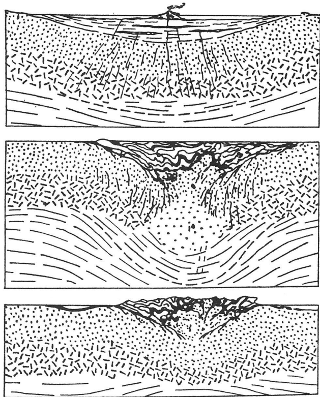
図7 地向斜造山運動の模式的過程 上:地向斜初期,中:造山期初期, 下:造山期末期。(山下昇,1967, 新版地球科学序説,築地書館。
