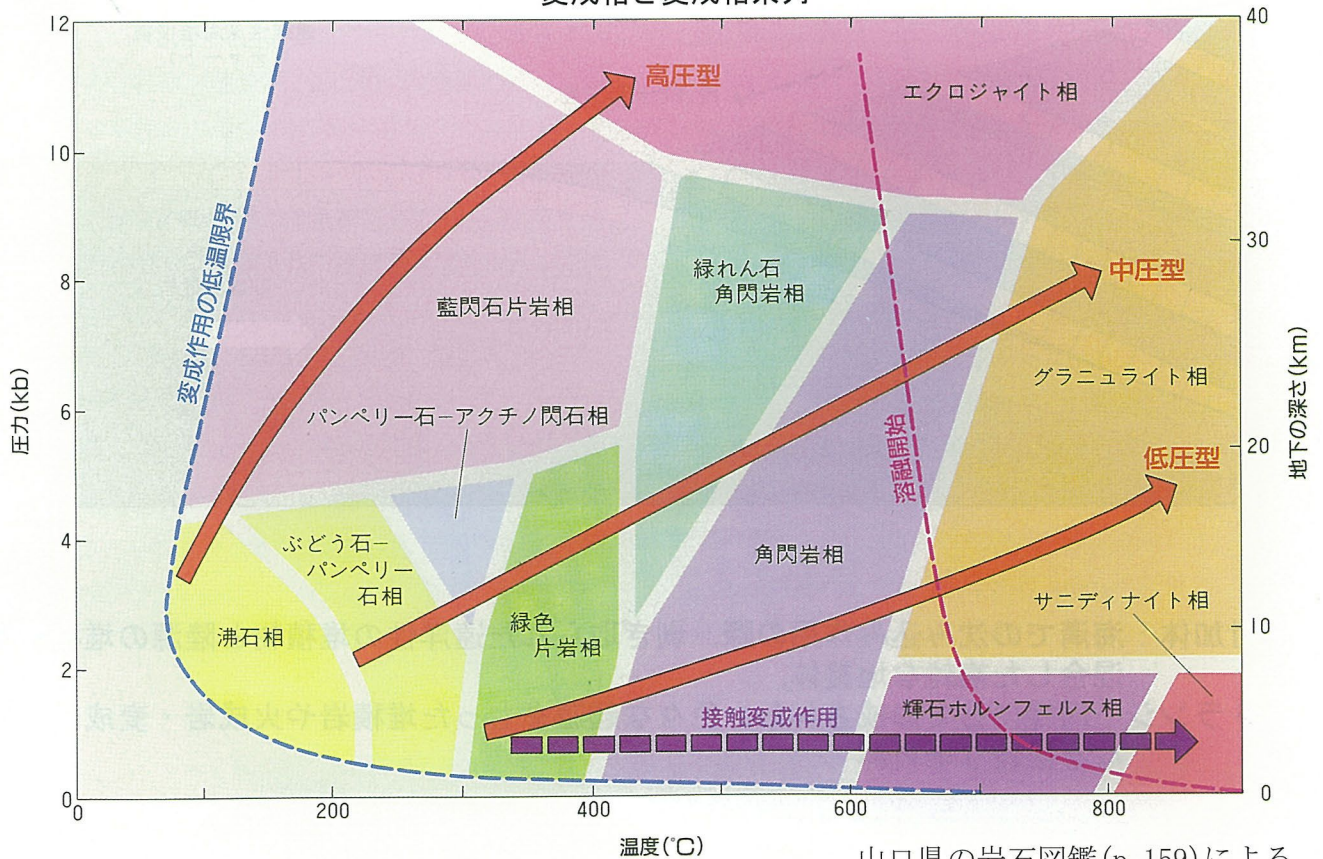
変成相と変成相系列
