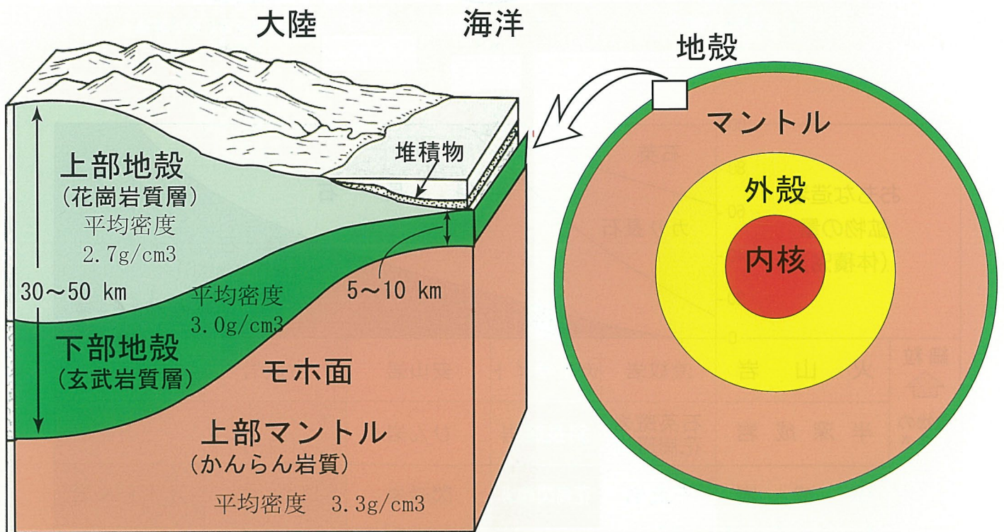
付図 1 地球の構造・地殻の構造
