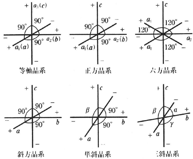
図 3.6 6つの結晶系 (三方晶系は広義の六方晶系に含む) 等軸晶系では3本の結晶軸の方向が同じ性質をもっているの で、 a, b, c としないで a_1, a_2, a_3 と書く。正方晶系でも a 軸と b 軸が同じ性質をもっているの、 a_1 と a_2 で示す。六方 晶系だけは4本の結晶軸をもちい、 c 軸に直交する平面上の 3本の結晶軸が同じ性質をもつので、 a_1, a_2, a_3 で示す。
