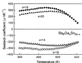
図1 ゼーベック係数の温度依存性
